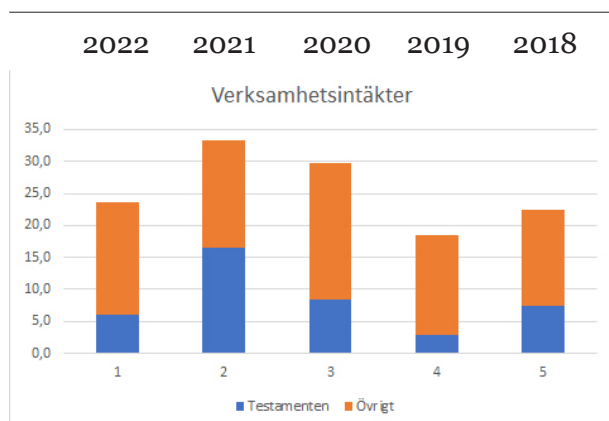
Verksamhetsintäkter 2018 - 2022, Mkr
